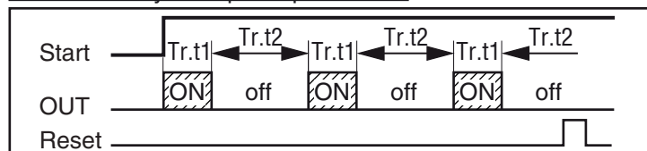
Oscillateur asymétrique départ à ON.
