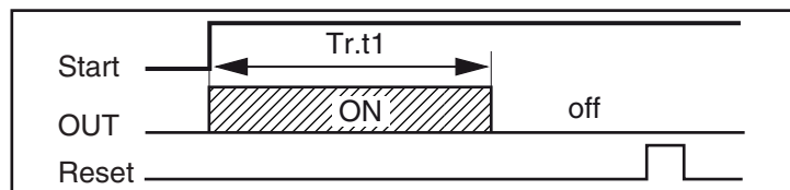
Oscillateur asymétrique départ à OFF.
